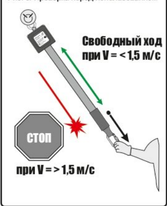
Рис. 10. Вытягивание и втягивание троса
