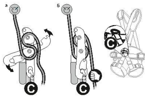
Рис. 6. Функционирование устройства
