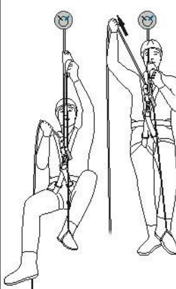
Рис. 13. Подъем с использованием зажима со стреленом
