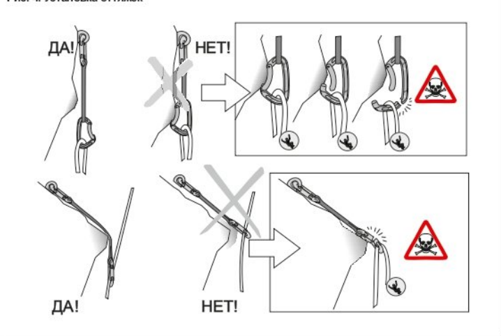
Рис. 5. Использование карабинов
