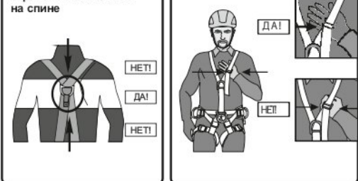
Рис. 10. Страховочная система
